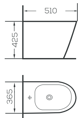
ESQUEMA (mm)
